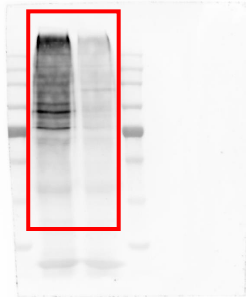
Immunoblot: HA
