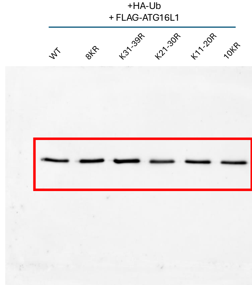
Immunoblot: FLAG
