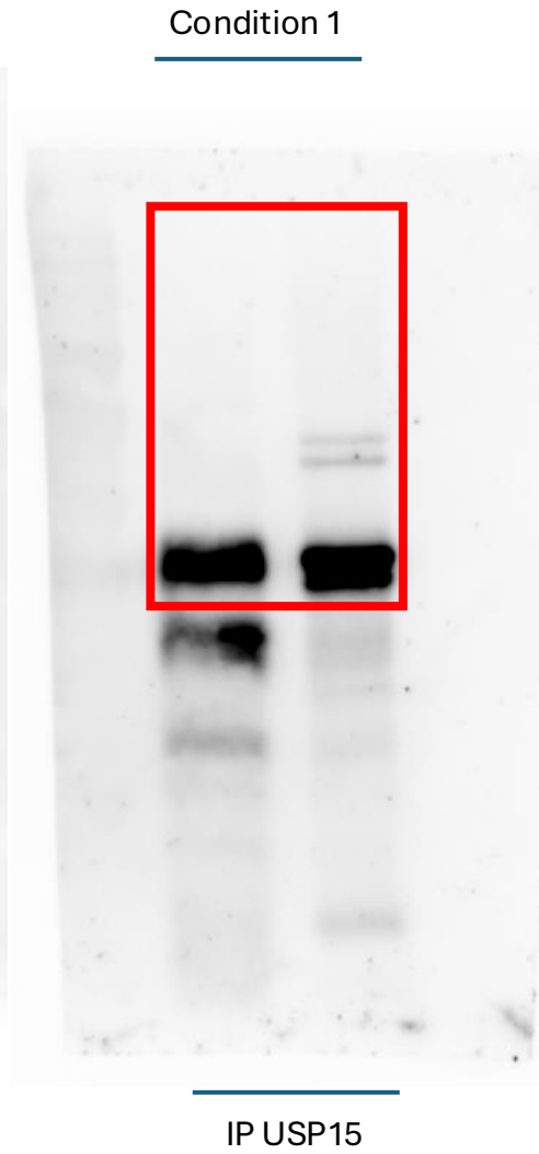
Immunoblot: Atg16l1
