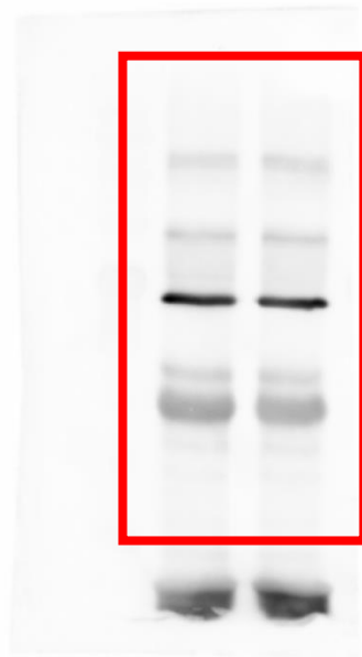
Immunoblot: FLAG
