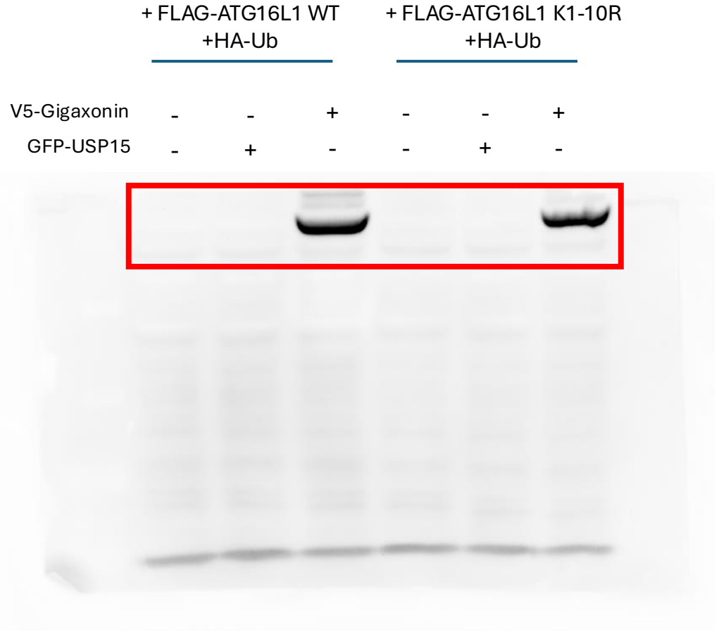
Immunoblot: V5
