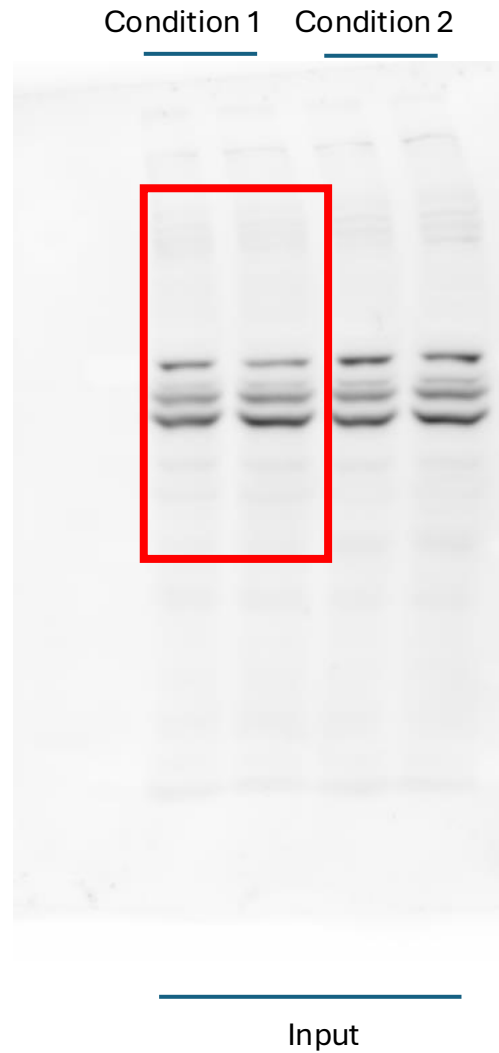
Immunoblot: Atg16l1
