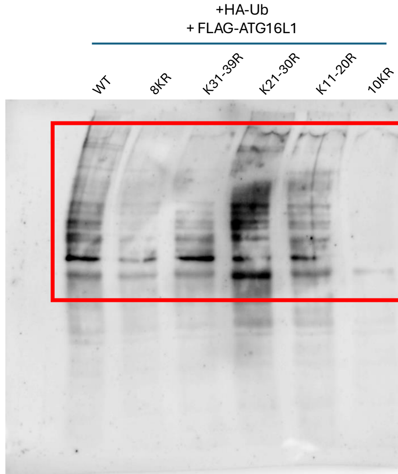
Immunoblot: HA
