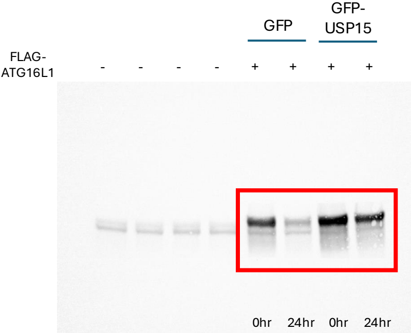
Immunoblot: FLAG
