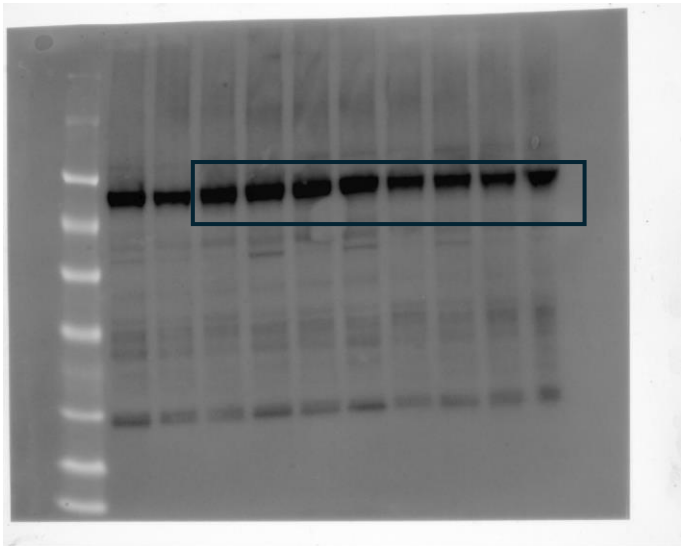
IB: Akt
