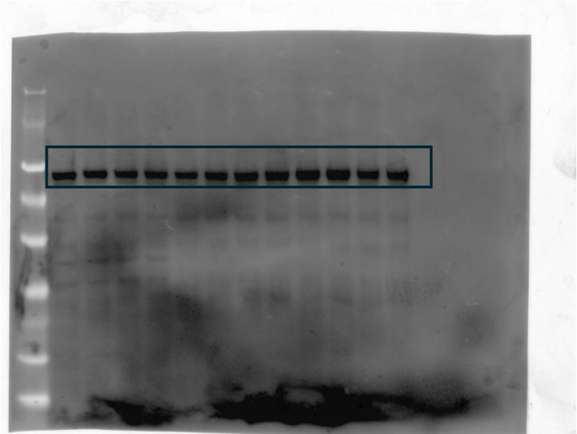
IB: Akt
